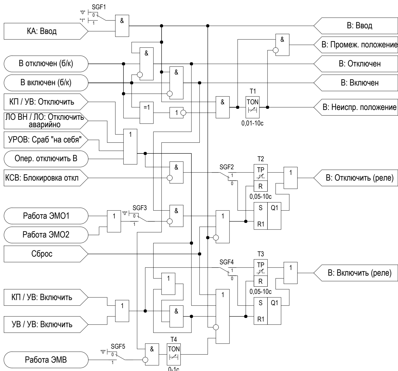
Рисунок 2.13 – Функциональная схема «Выключатель»
