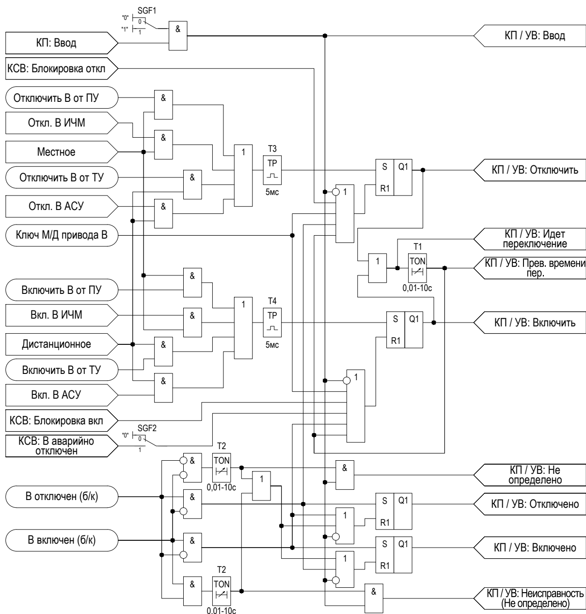
Рисунок 2.11 – Функциональная схема «УВ»
